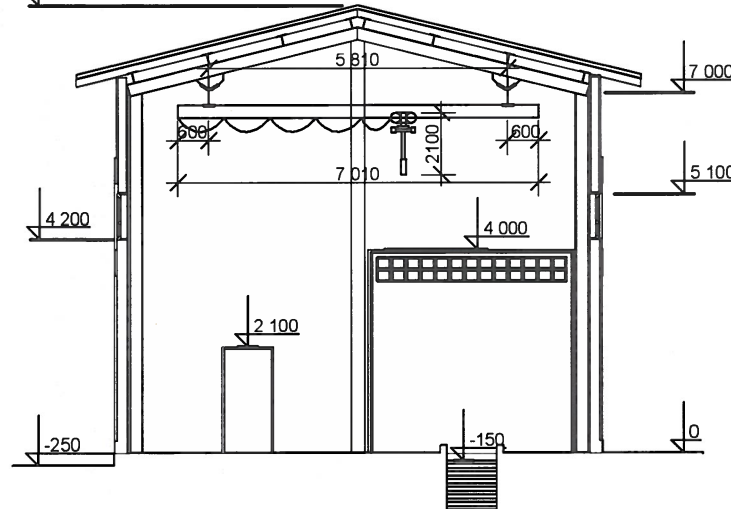
Sectiunea 2-2
